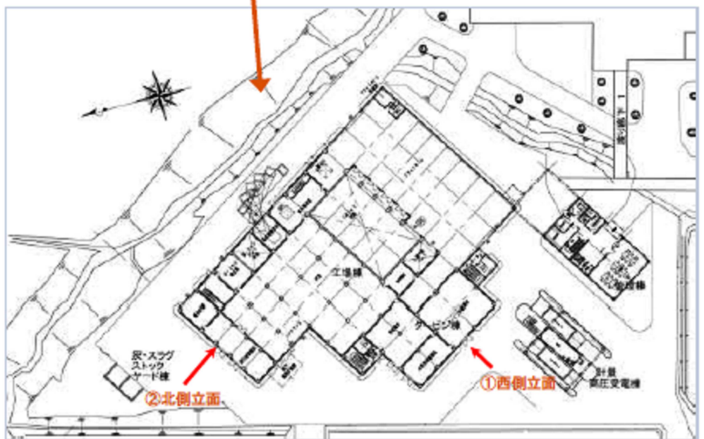
新焼却施設配置計画 (案)
